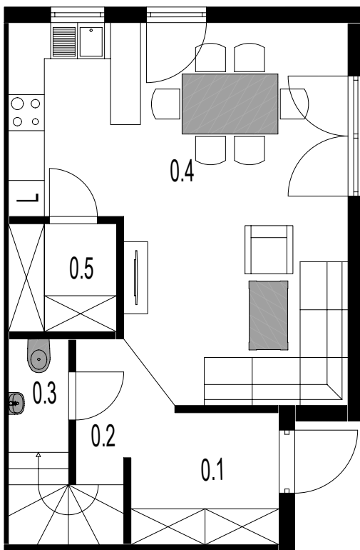
Rzut parteru
