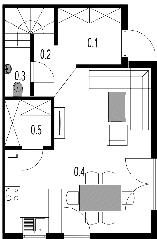
Rzut parteru
